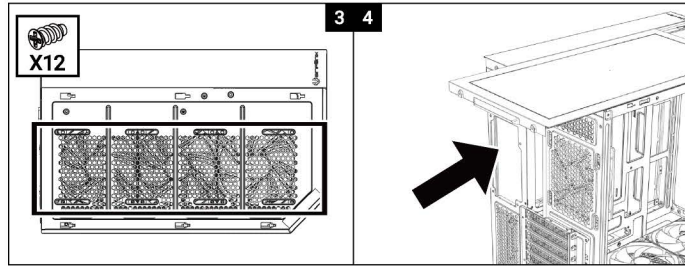
Fan (Bottom) Installation/Installation du ventilateur inférieur 風扇(底部)安裝/風扇(底部)安装
