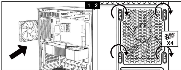
MB Tray Installation/Installation du ventilateur avant 風扇(前方)安裝/風扇(前方)安装
