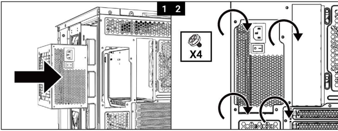
Fan (Back) Installation/Installation du ventilateur arrière 風扇(後方)安裝/風扇(后方)安装
