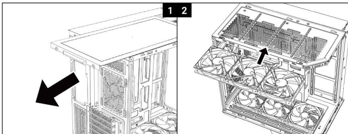
Fan (Top) Installation/Installation du ventilateur supérieur 風扇(上方)安裝/風扇(上方)安装
