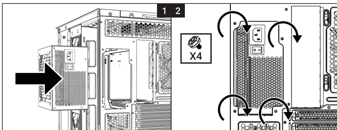
Fan (Back) Installation/Installation du ventilateur arrière 風扇(後方)安裝/風扇(后方)安裝
