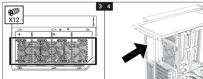
Fan (Bottom) Installation/Installation du ventilateur inférieur 風扇(底部)安裝/風扇(底部)安裝
