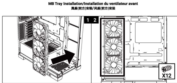
MB Tray Installation/Installation du ventilateur avant 風扇(前方)安裝/風扇(前方)安裝
