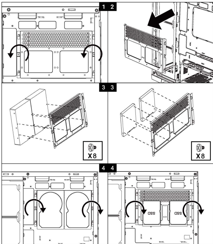
PSU Installation/Installation du bloc d'alimentation/電源安裝/电源安装
