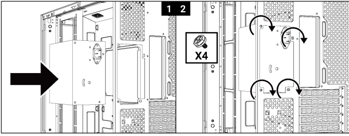
Fan (Back) Installation/Installation du ventilateur arrière 風扇(後方)安裝/風扇(後方)安裝 / Fan Montajı (Arka)
