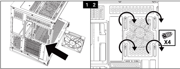
MB Tray Installation/Installation du ventilateur du plateau de la carte mère 風扇(主板)安裝/風扇(主板)安裝/Fan Montajı (MB Tray)
