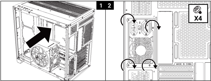
Fan (Back) Installation/Installation du ventilateur arrière 風扇(後方)安裝/風扇(后方)安裝/Fan Montajı (Arka)
